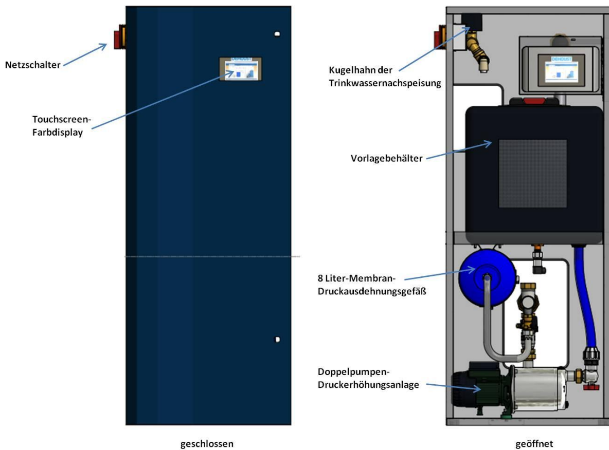
Abbildung 2: Aufbau der C-Class CONNECT : Vorderseite
